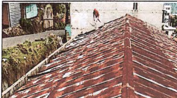
Foto 4: sustitución de lamina, por lámina troquelado aluzinc calibre 26
